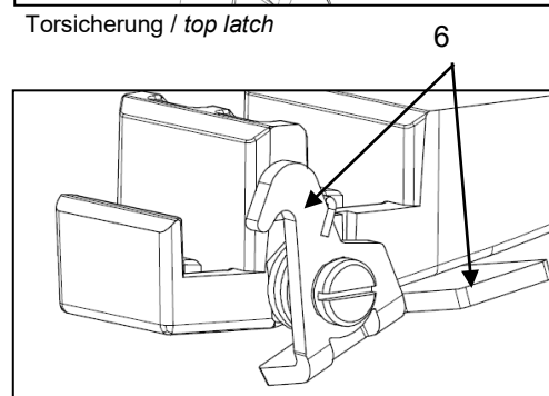
Zweite Torsicherung / second barndoor catch
